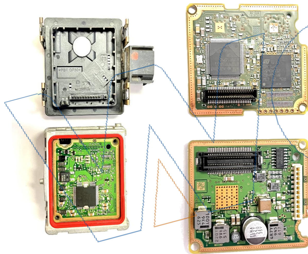
雷达组成
