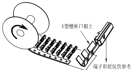
端子电镀后绕盘方向示意图
