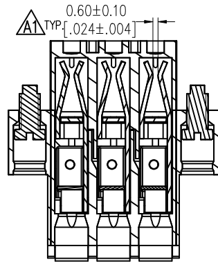
SEC A-A
